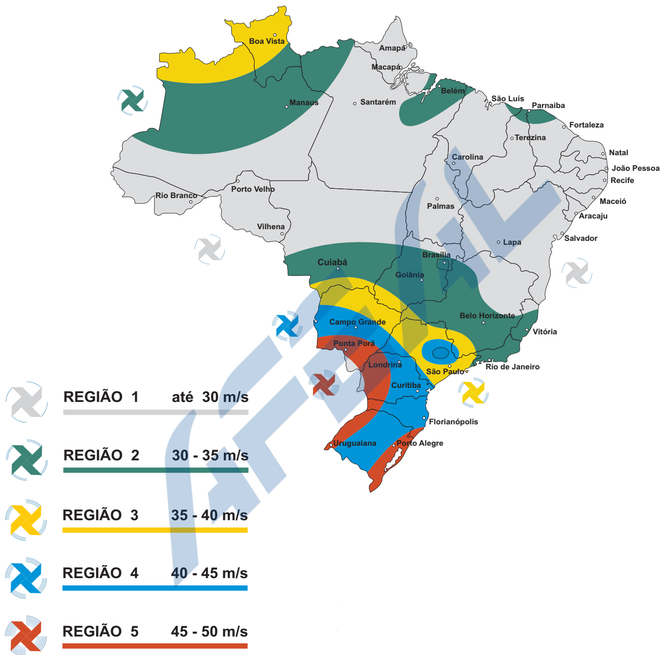
Mapa de isopletas ABNT NBR-6123
